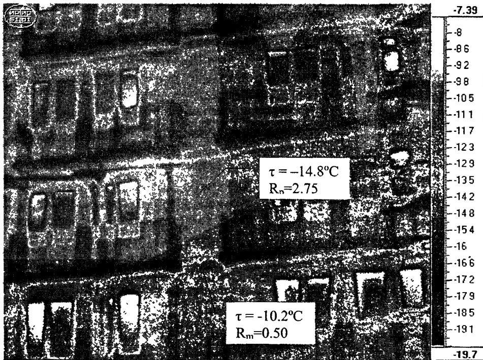
Рис.4. Составление термограммы
